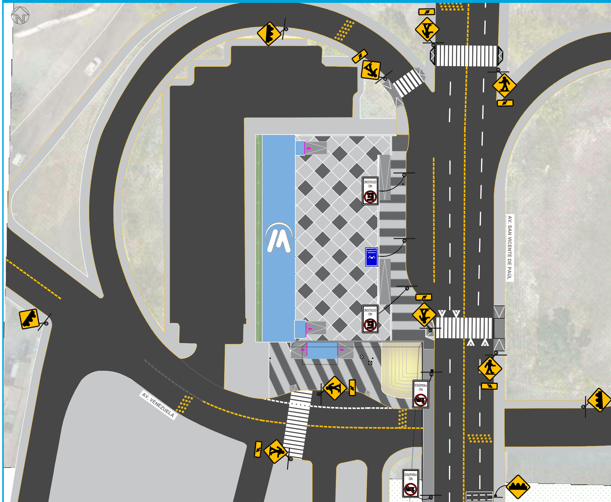
DETALLE 1: ESPACIAMIENTO DE BANDAS SONORAS
