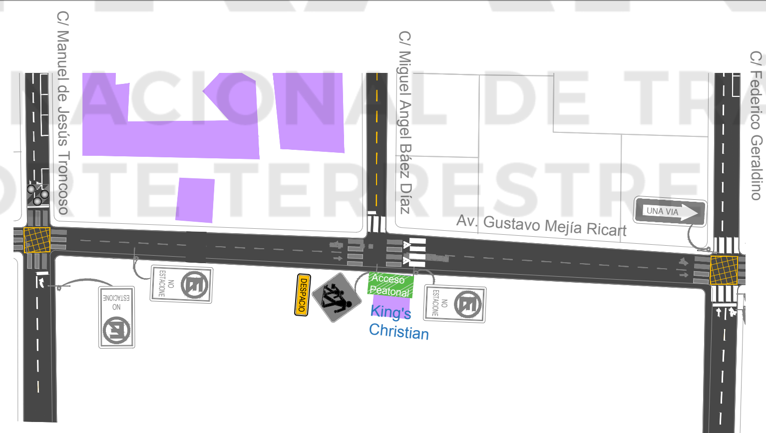
4 Señalización Propuesta King's Christian A-8
