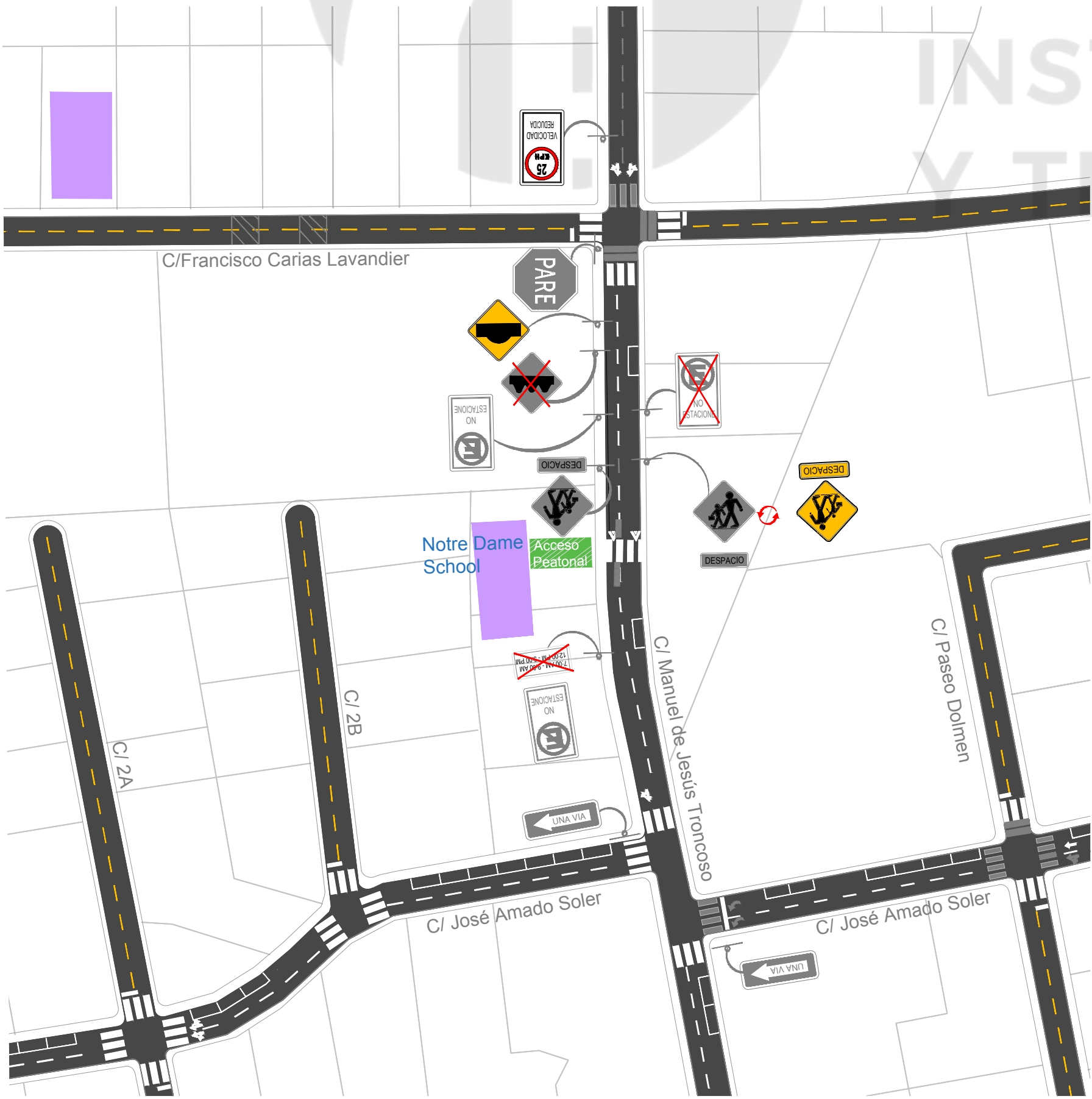
3 A-7 Señalización Propuesta Notre Dame School
