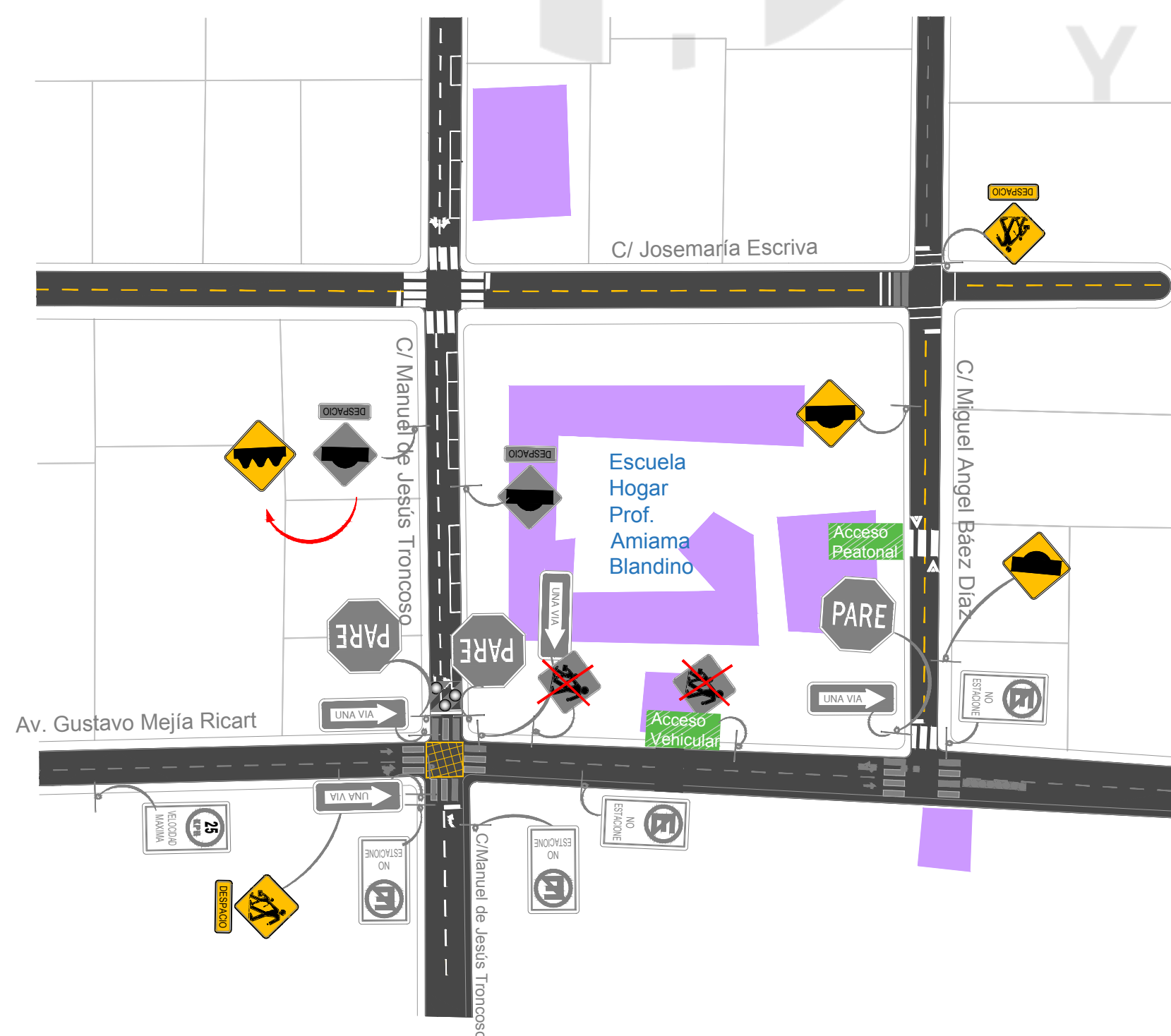
3 Señalización Propuesta Escuela Hogar Prof. Amiana Blandino A-8
