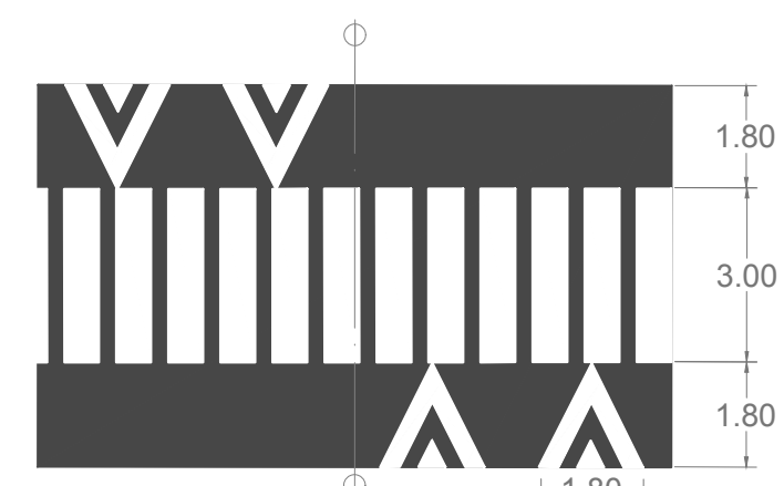
5 Detalle en planta reductor de velocidad (Speed Hump) A-8
