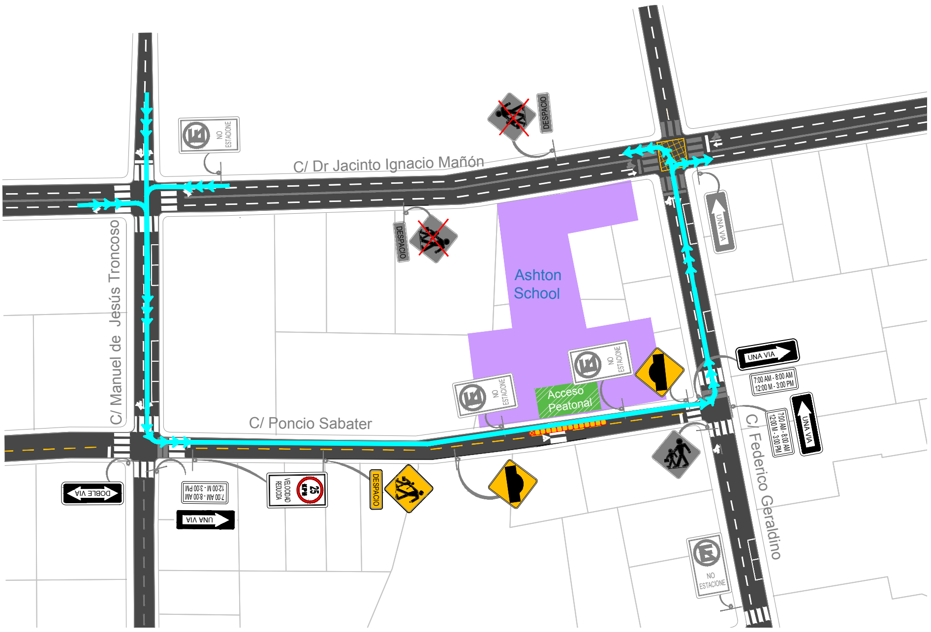
1 A-7 Señalización Propuesta Ashton School
