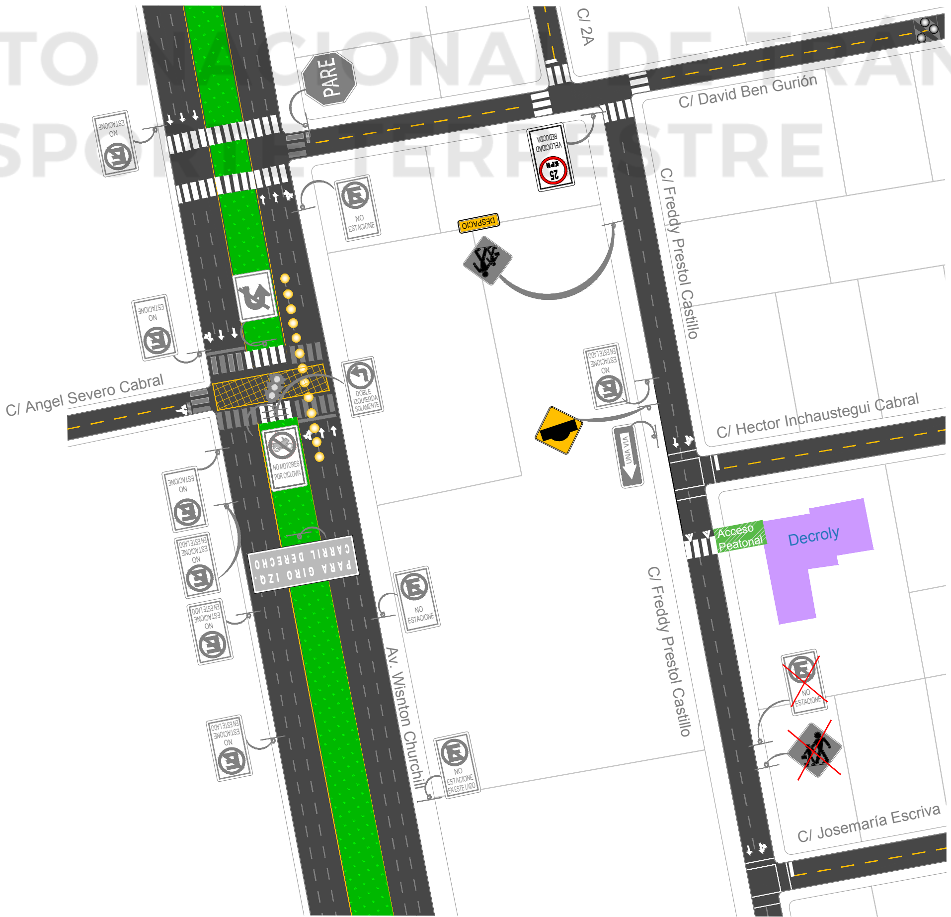
4 A-7 Señalización Propuesta Decroly
