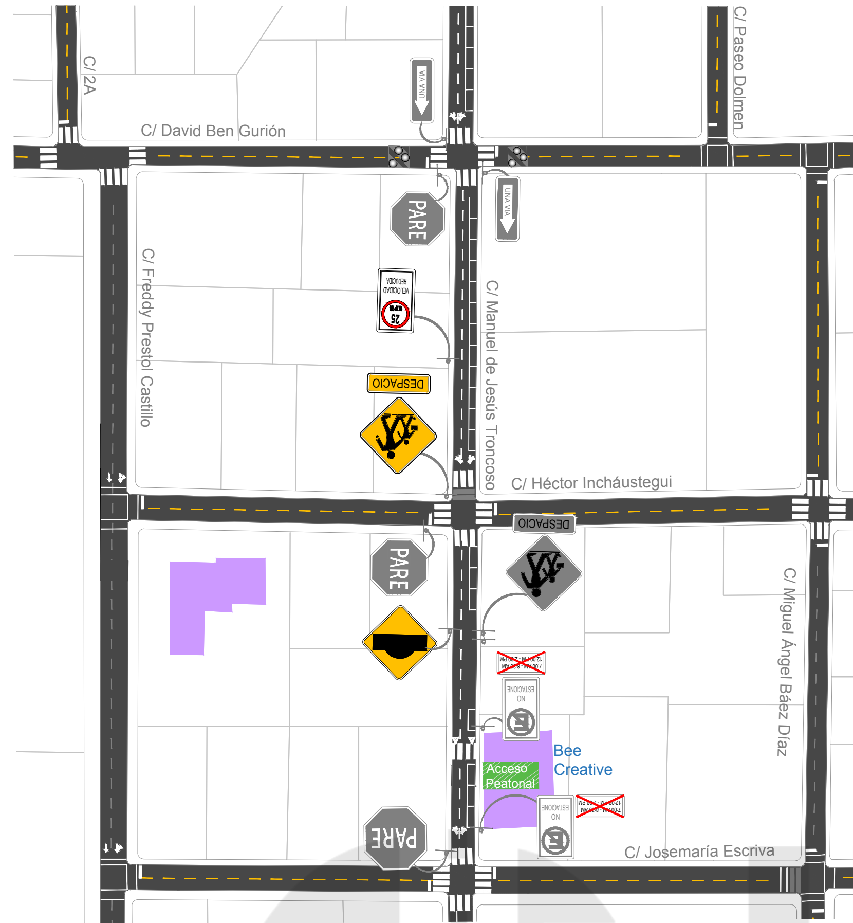
1 Señalización Propuesta King's Christian A-8
